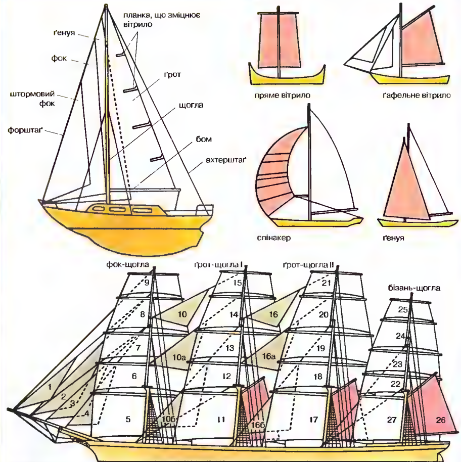
Розташування вітрил
